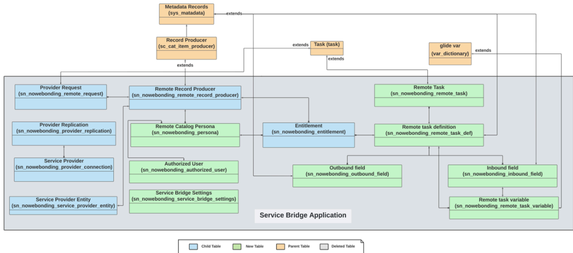
서비스 브리지 고객 데이터 모델
